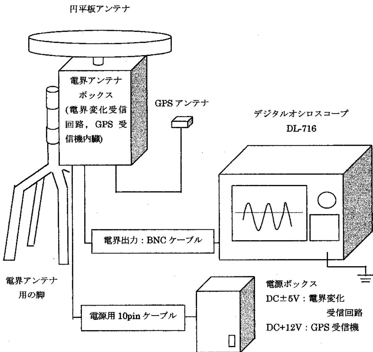
図1-1. 電界アンテナ観測装置概略図
