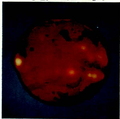
— 22 GHz — 02 H 47 M UT
