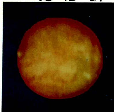
— 90 GHz — 03 H 13 M UT
