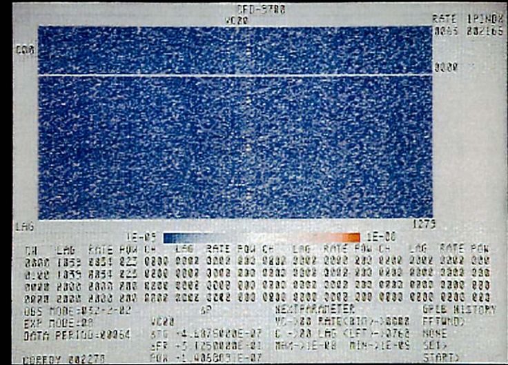
W49N (H 2 O maser)
